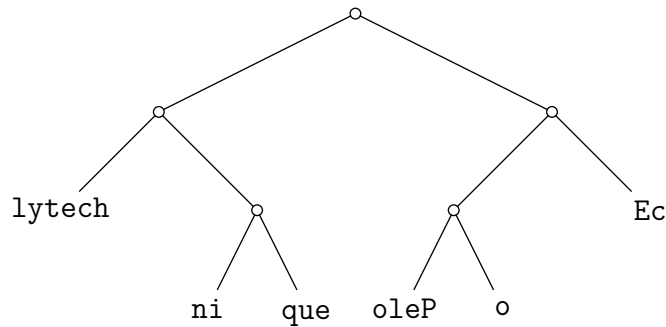
Figure 2 Après la phase 1
