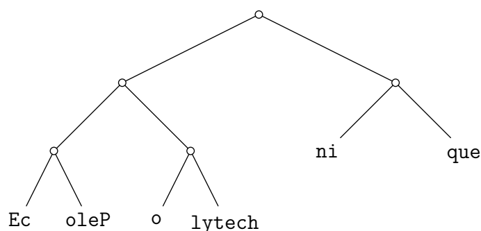
Figure 1 La corde obtenue par l'algorithme
