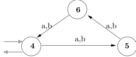
Automate A_{2\_ex}
