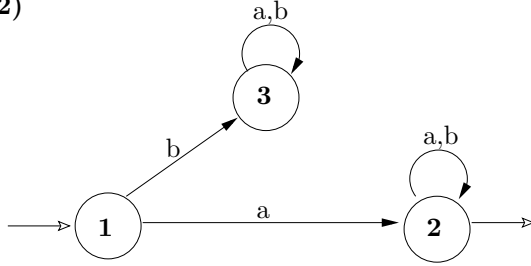
Automate A_{1\_ex}
