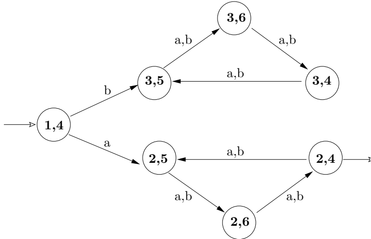
Automate A_{3\_ex}
